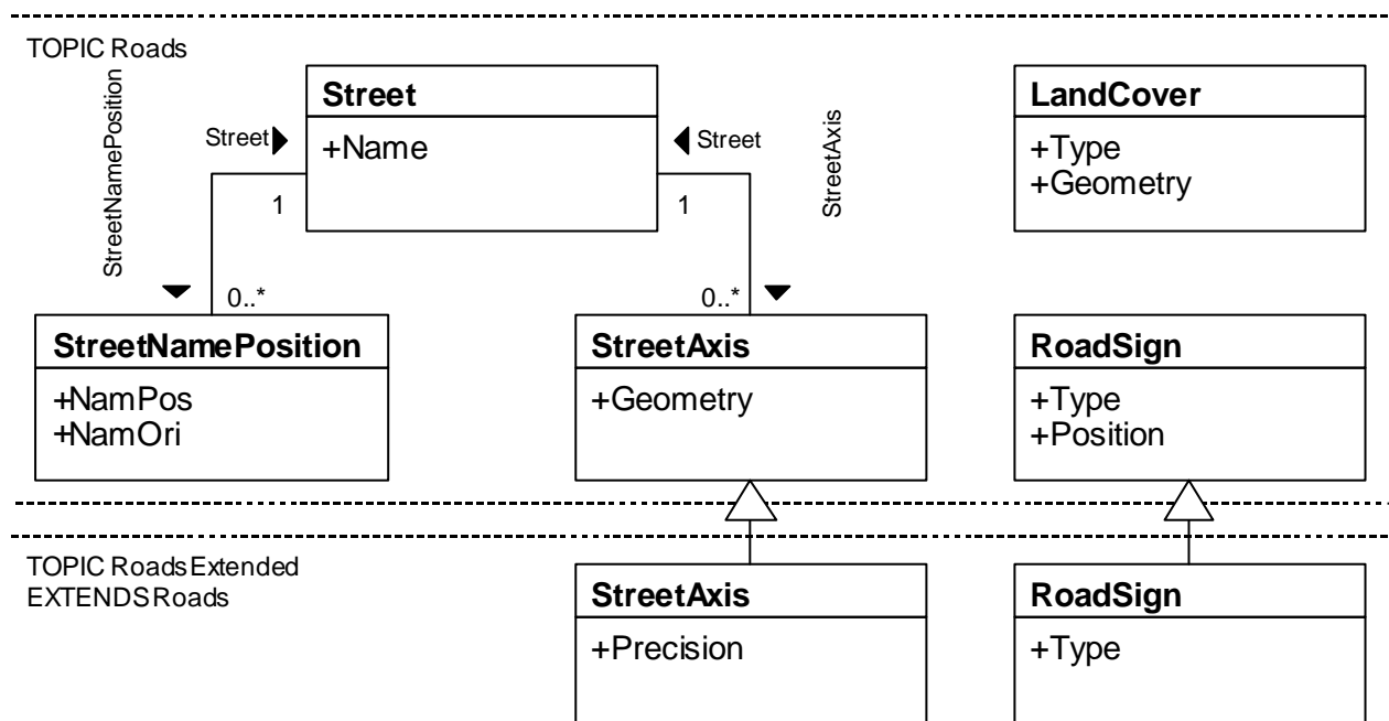
Figure 26 : Modèle conceptuel UML du "petit exemple Roads".
